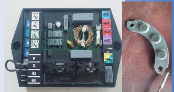
Automatic Voltage Regulator (AVR) dan diode untuk berbagai merk dan tipe generator
