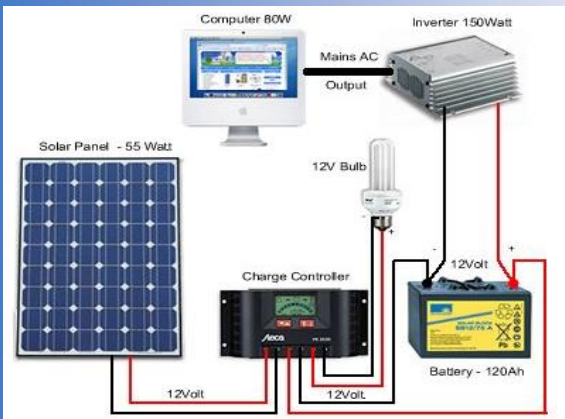
Listrik tenaga surya untuk skala rumah tangga (Off grid)
